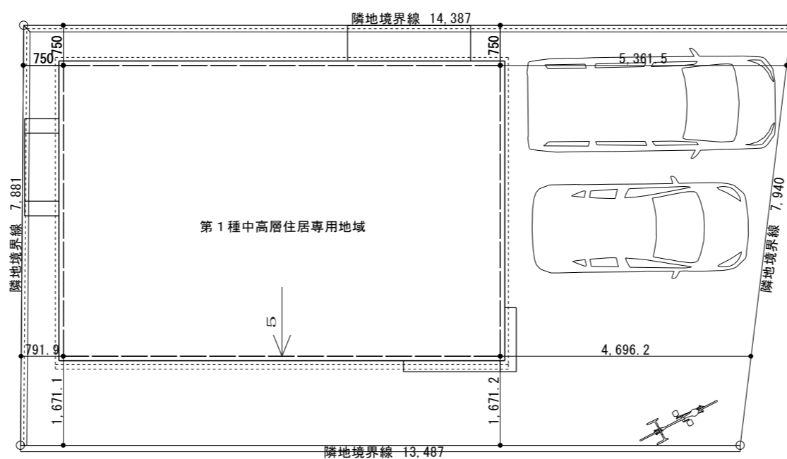
配置図 S=1/100
