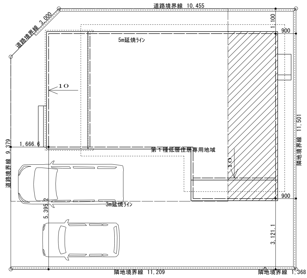
配置図 S=1/100
