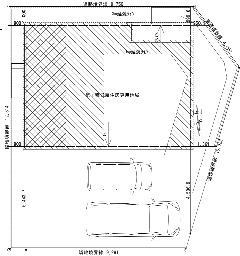
配置図 S=1/100
