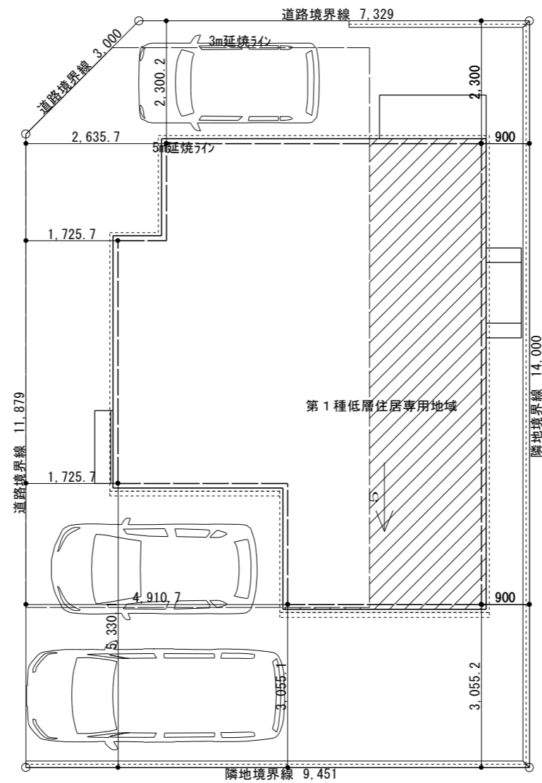
配置図 S=1/100
