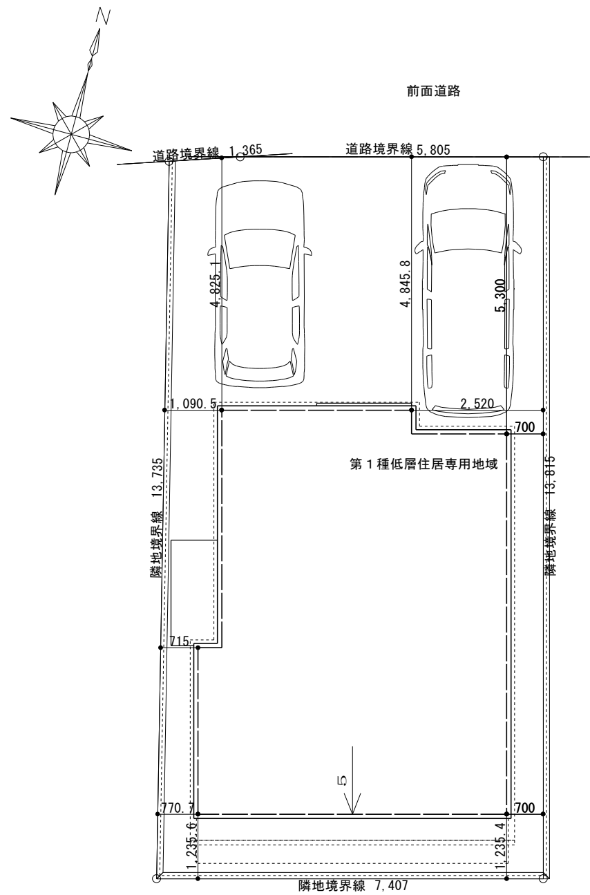
配置図 S=1/100
