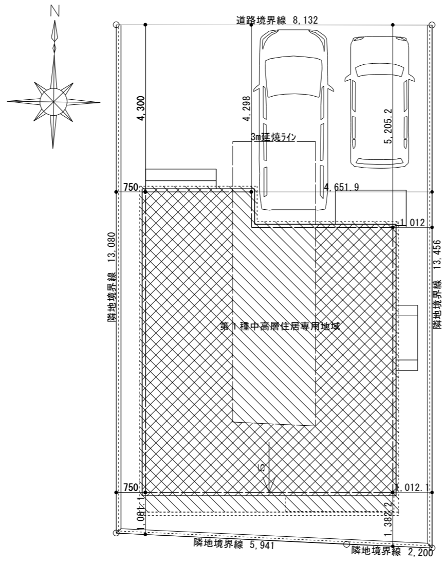
配置図 S=1/100
