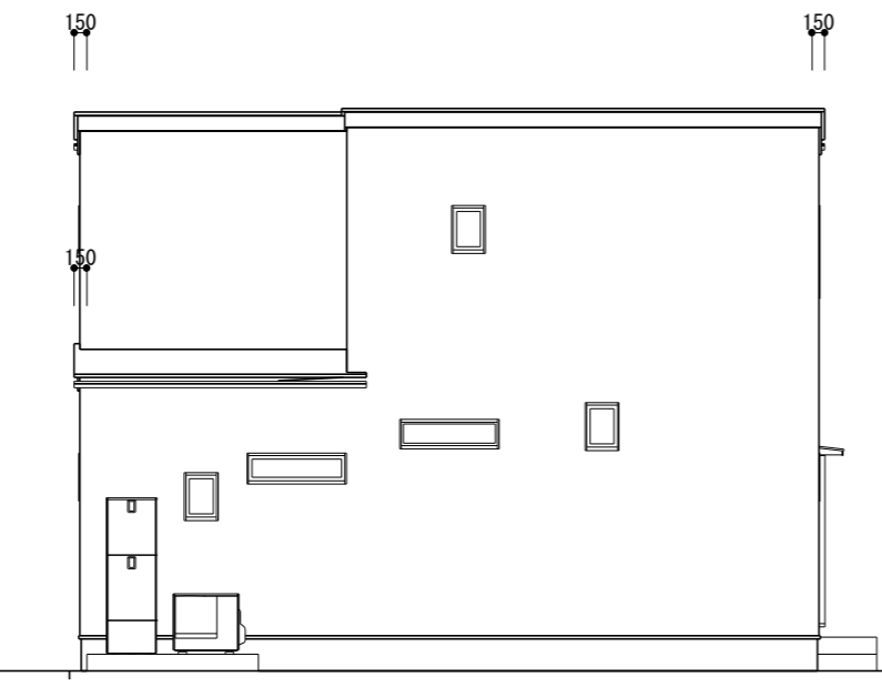
北立面図 S=1/100
