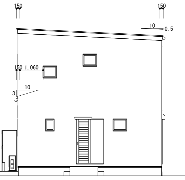
西立面図 S=1/100
