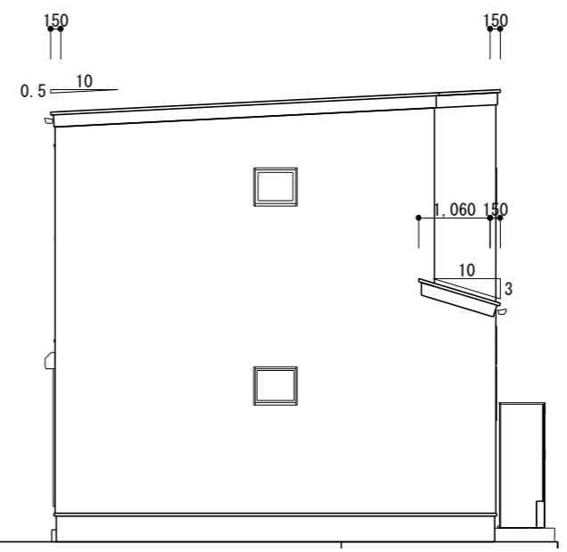
東立面図 S=1/100
