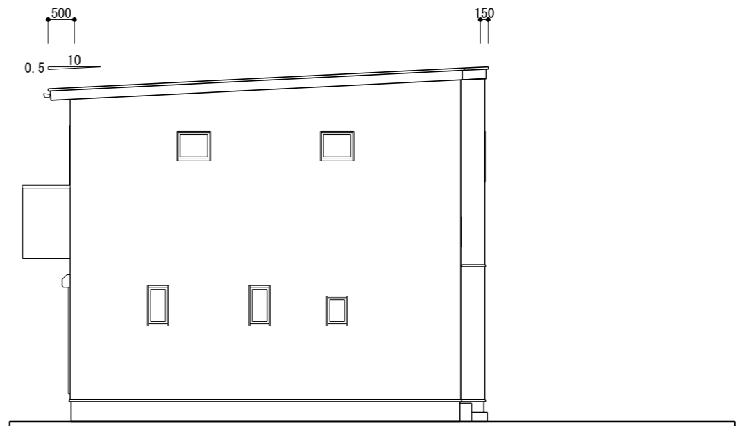
東立面図 S=1/100
