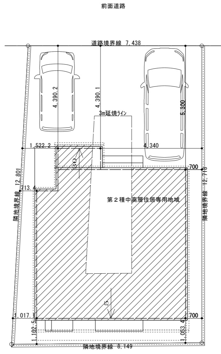
配置図 S=1/100
