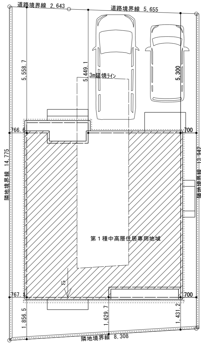
配置図 S=1/100
