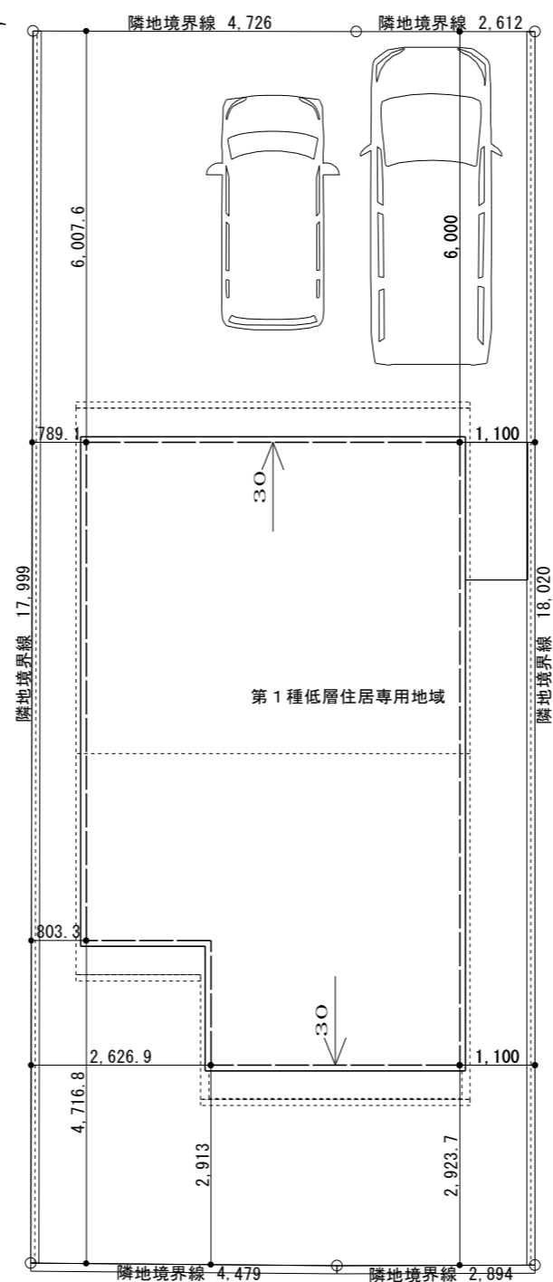
配置図 S=1/100
