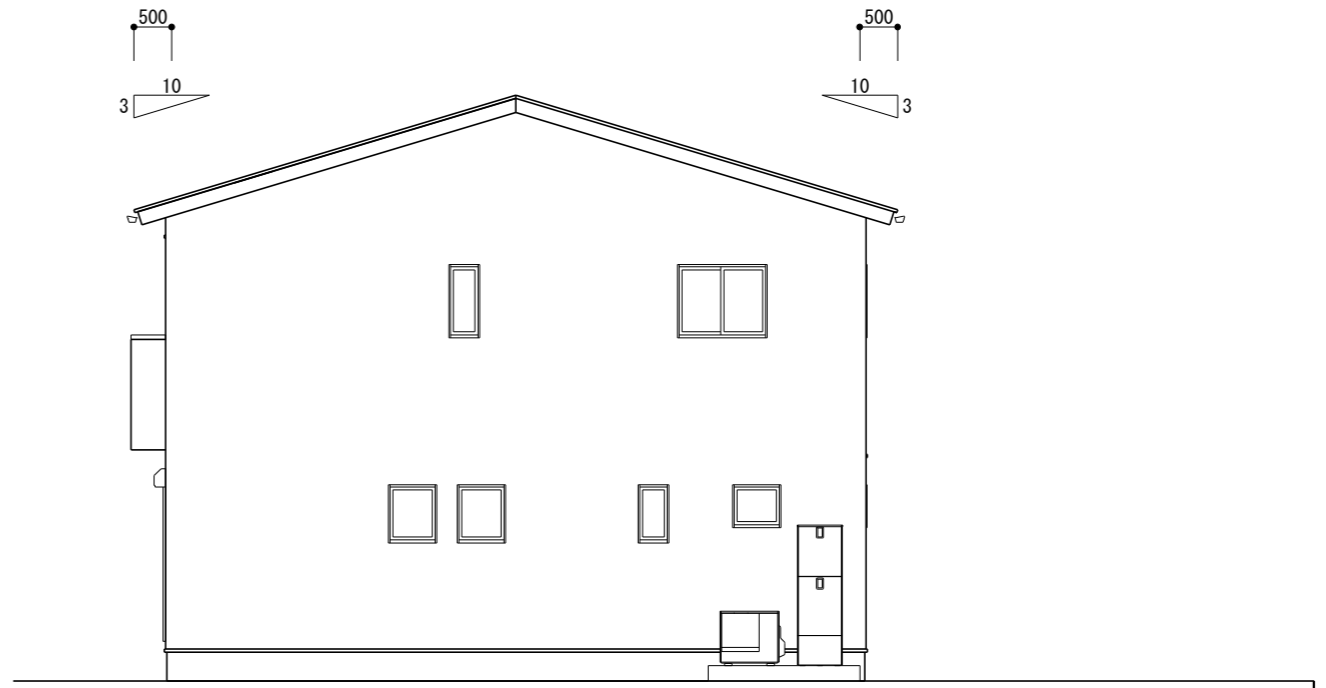
東立面図 S=1/100
