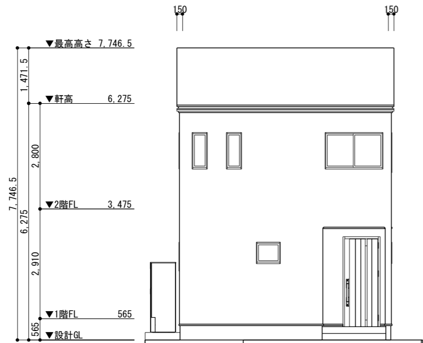
北立面図 S=1/100
