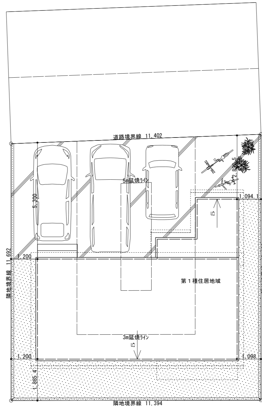
配置図 S=1/100
