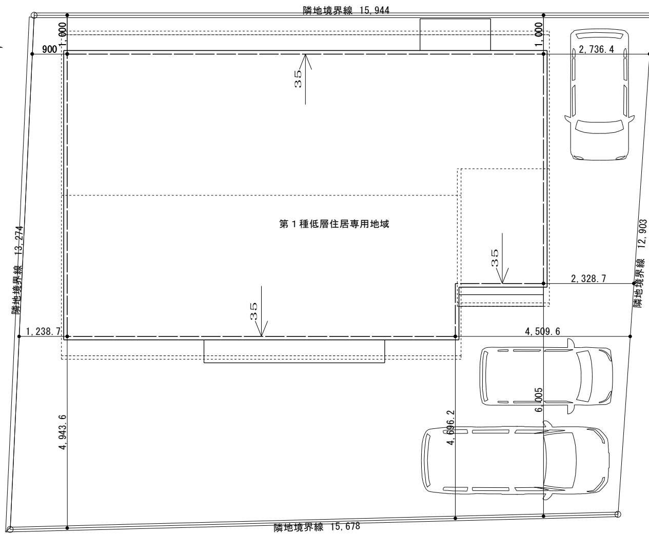
配置図 S=1/100
