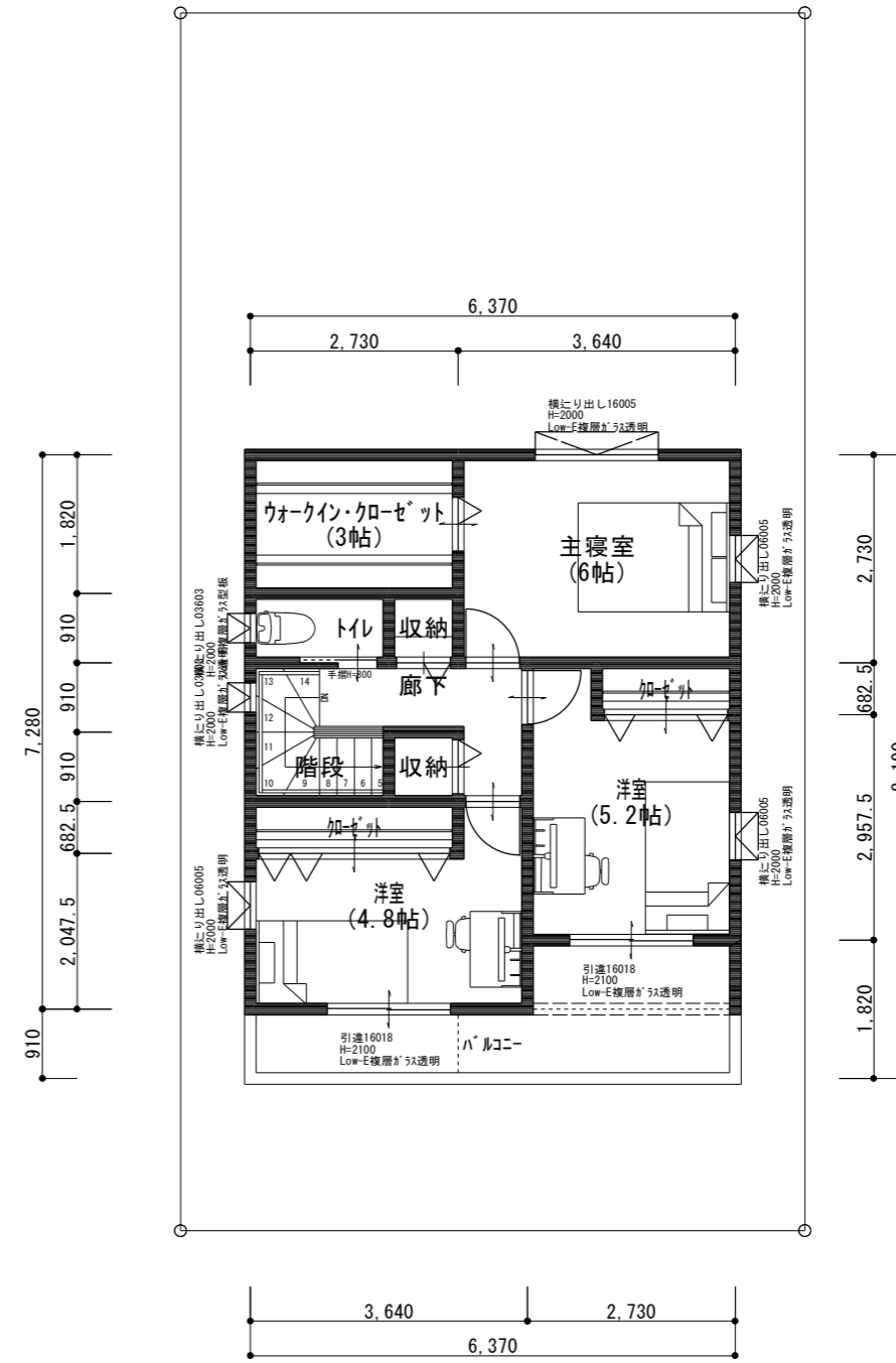
2階平面図 S=1/100
