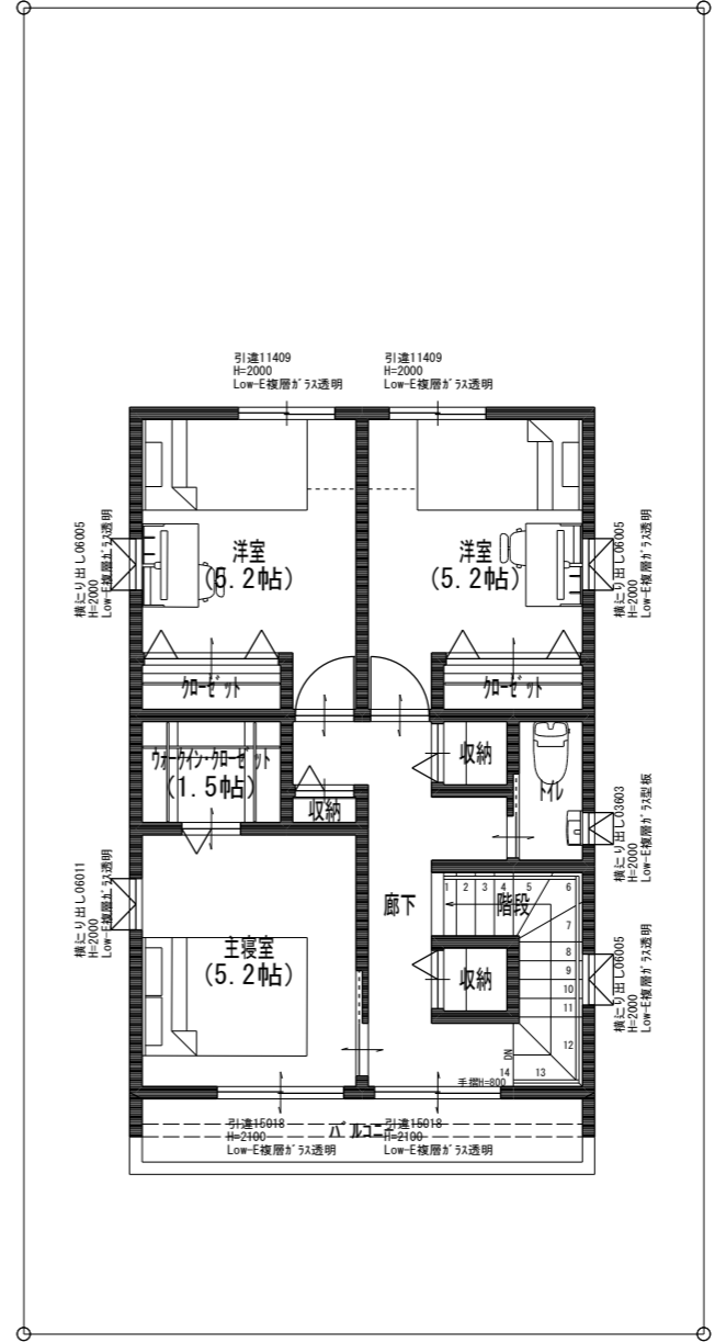
2階平面図 S=1/100
