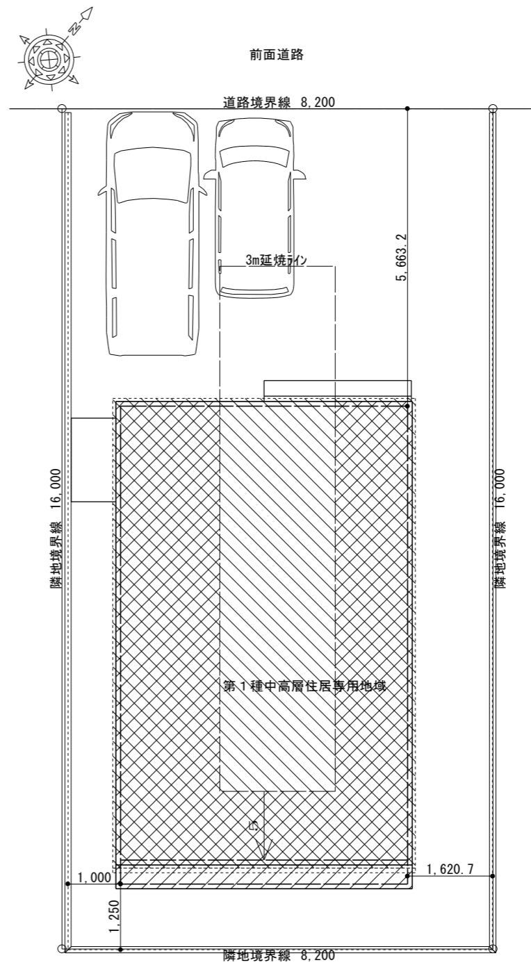
配置図 S=1/100
