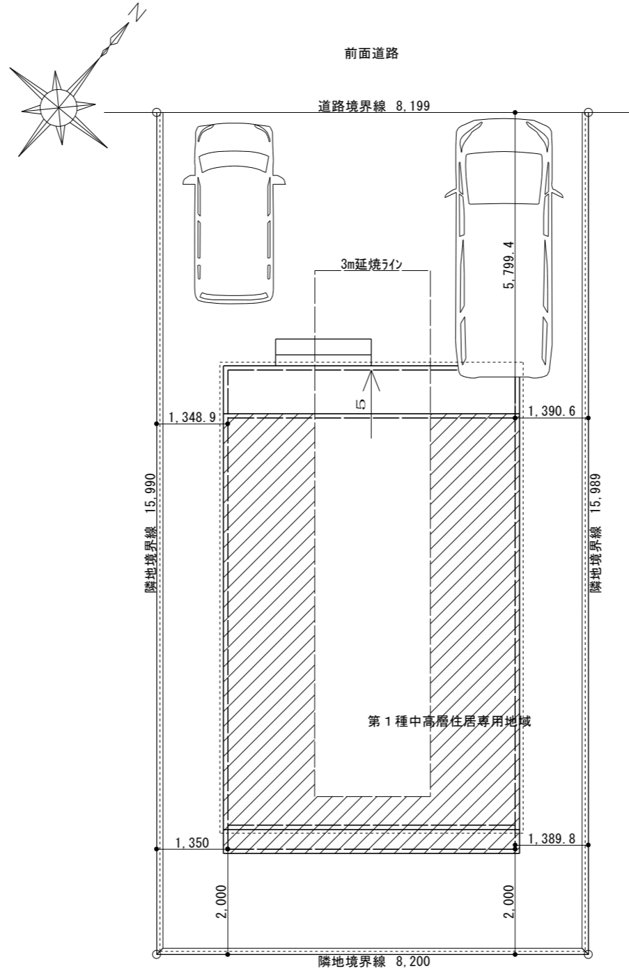
配置図 S=1/100
