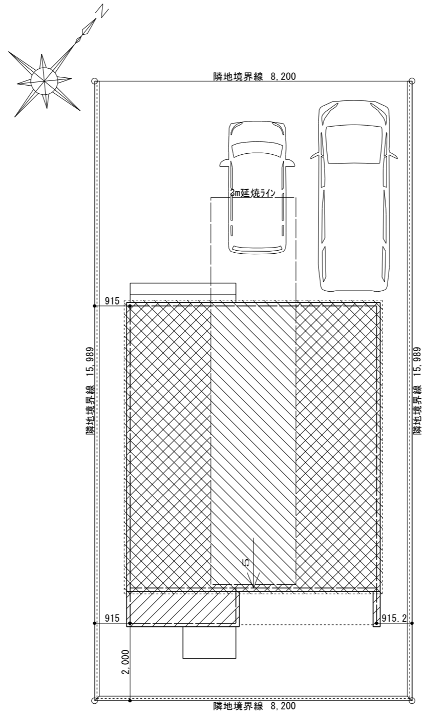
配置図 S=1/100
