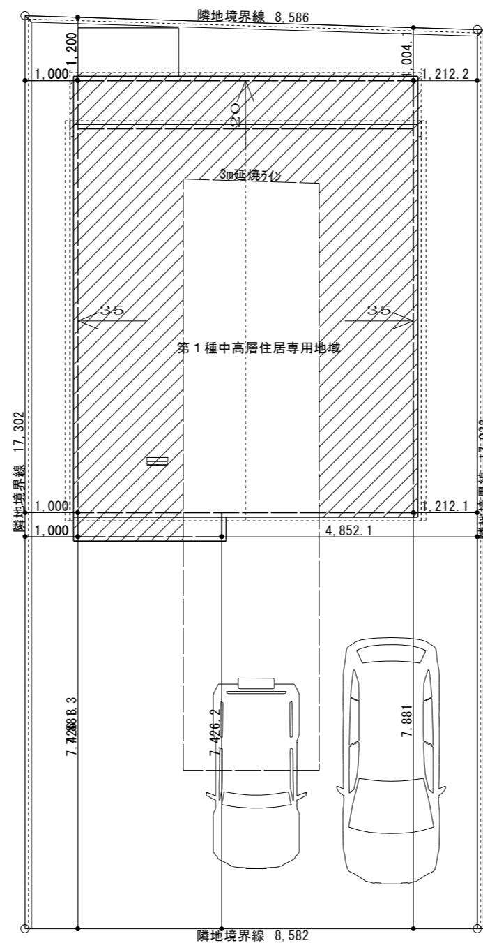
配置図 S=1/100
