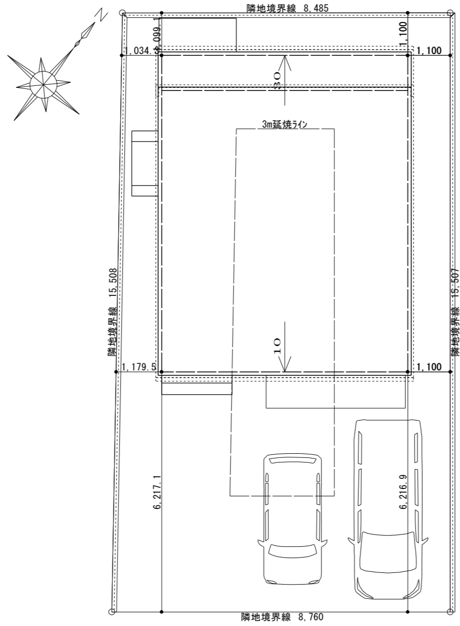
配置図 S=1/100
