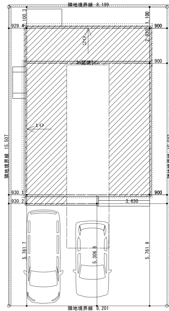
配置図 S=1/100
