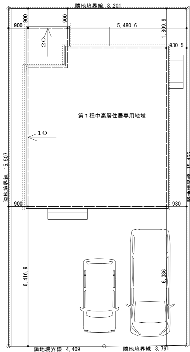
配置図 S=1/100
