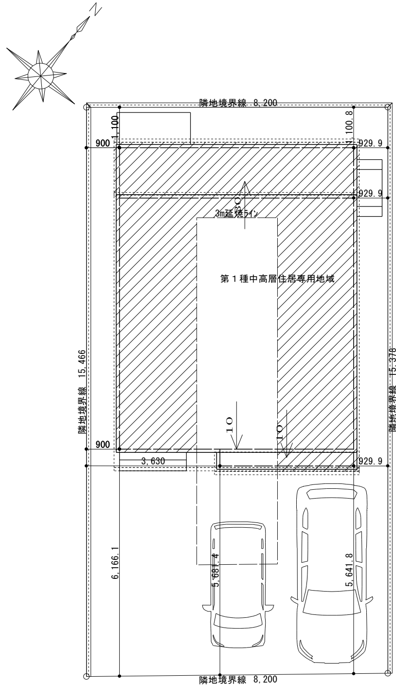
配置図 S=1/100
