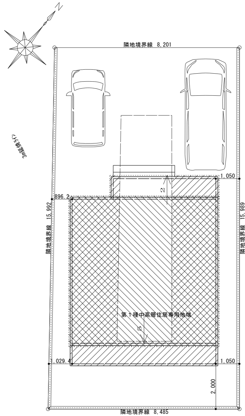
配置図 S=1/100
