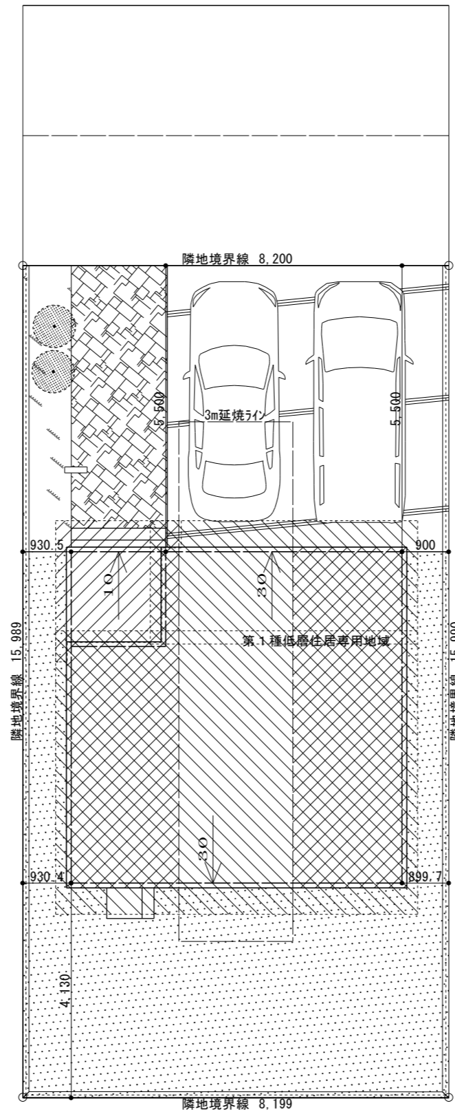
配置図 S=1/100
