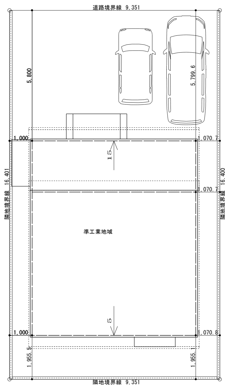
配置図 S=1/100
