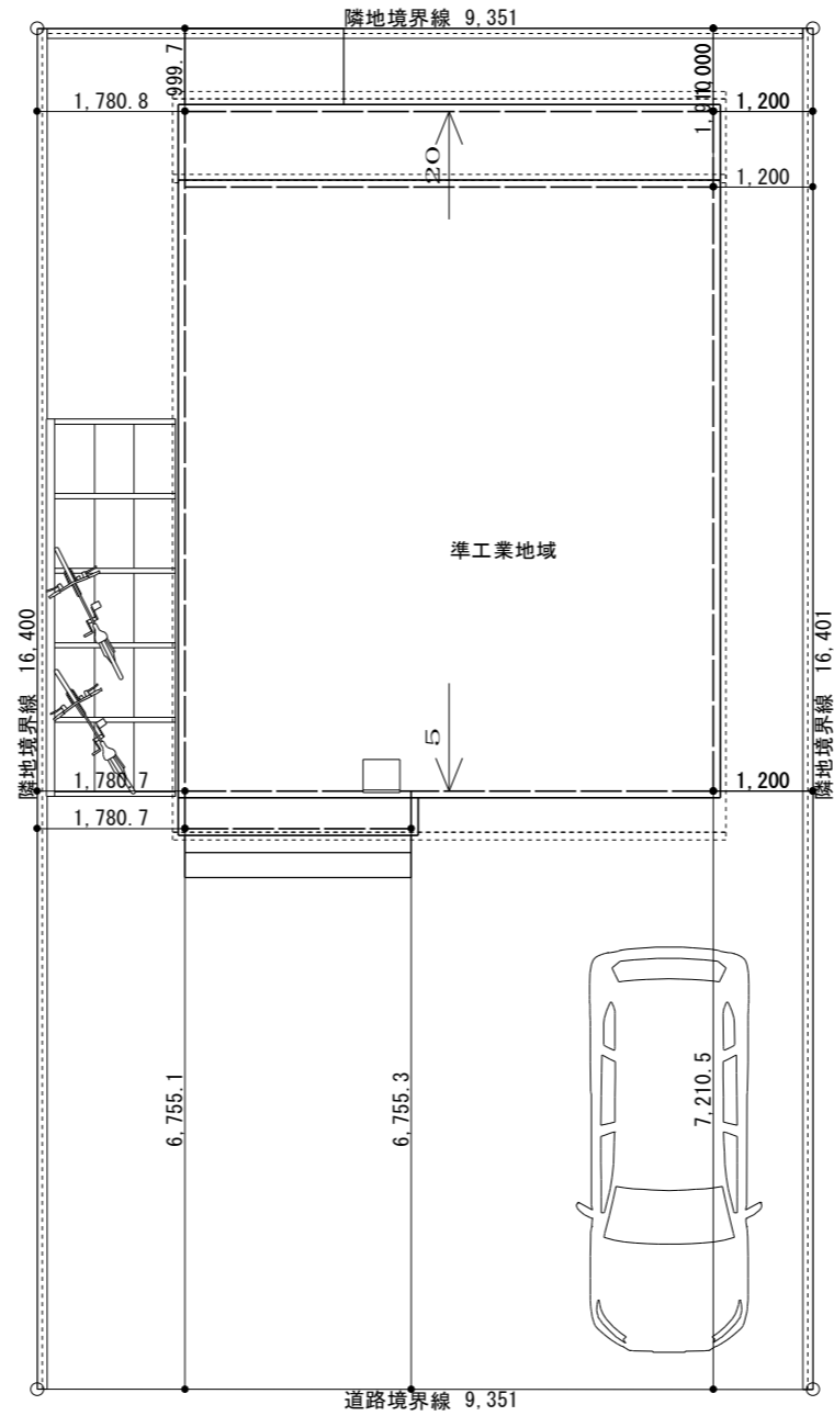
配置図 S=1/100
