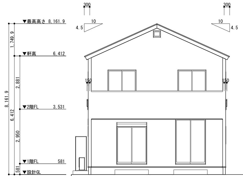
南立面図 S=1/100
