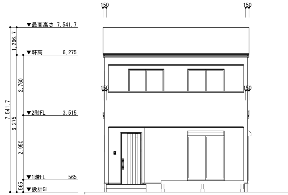
南立面図 S=1/100
