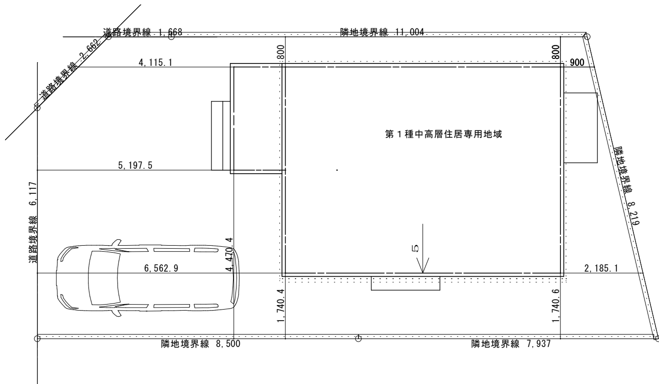
配置図 S=1/100
