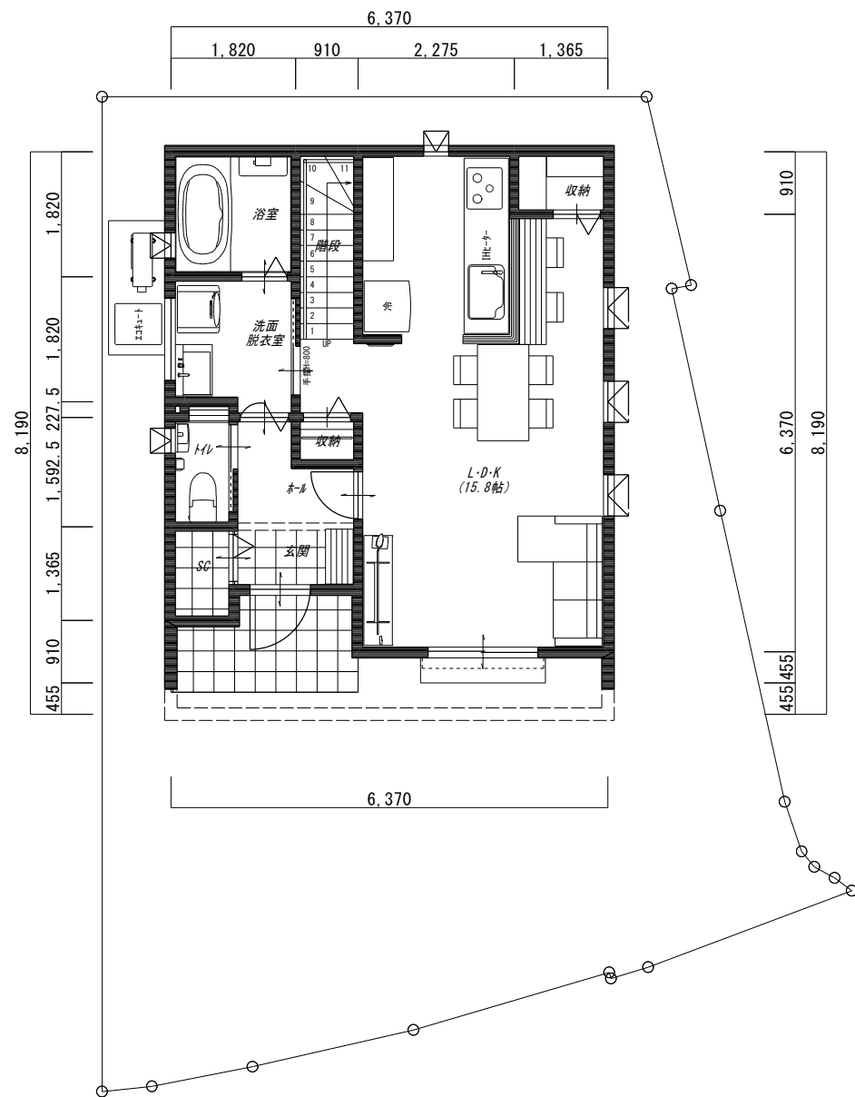
1階平面図 S=1/100
